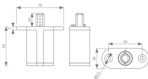
bovenste deel deur
