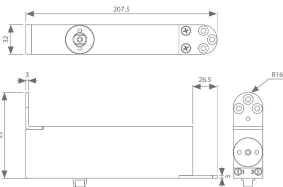
onderste deel deur - hoekpositie
