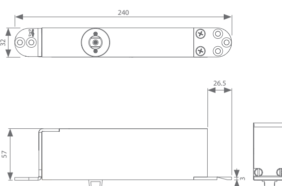
onderste deel deur - centrale of decentrale positie
