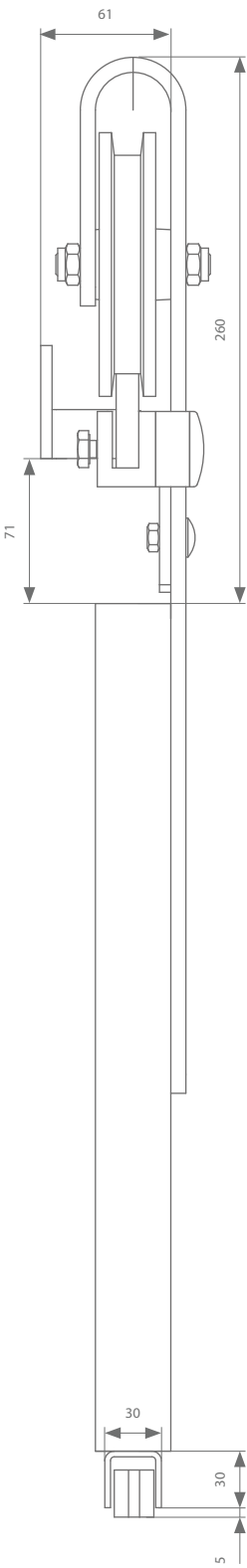
Vloergeleiding optie 1
