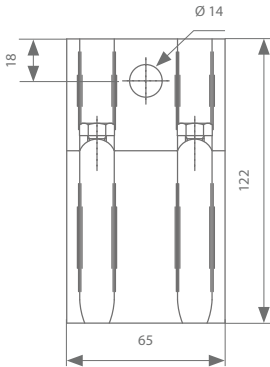
Verbindingsmuurbeugel 131.120 131.127 (inox)
