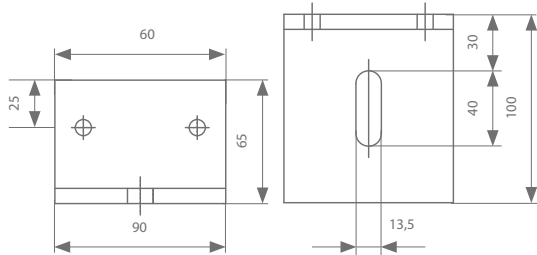
Draagstuk 131.910 131.917 (inox)
