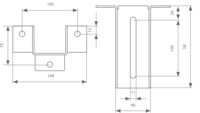
Dubbel draagstuk 121.930
