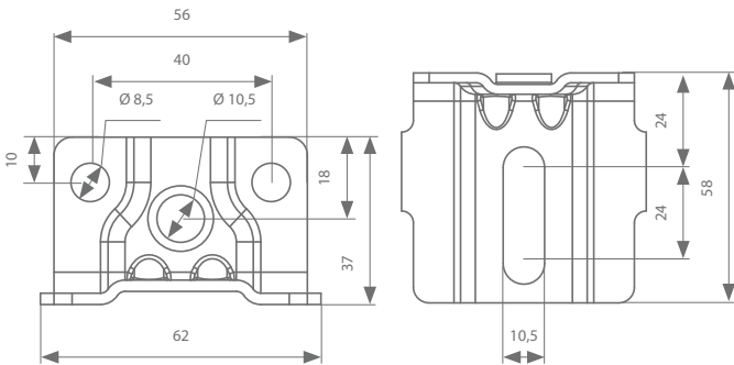
Draagstuk 121.910 121.917 (inox)
