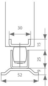
Vloergeleiding optie 2
