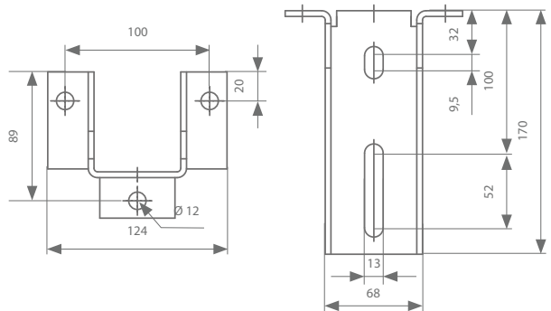
Dubbel draagstuk 131.930
