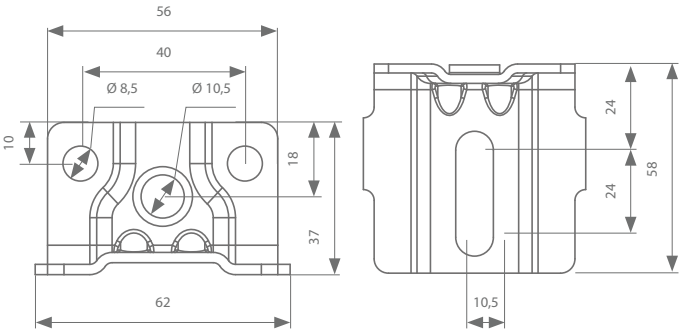
Draagstuk 121.910 121.917 (inox)
