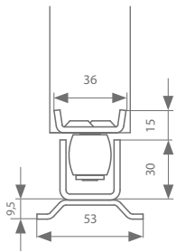
Vloergeleiding optie 2
