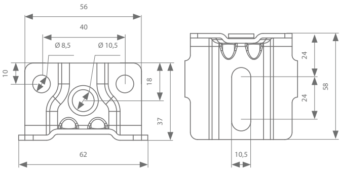
Draagstuk 121.910 121.917 (inox)
