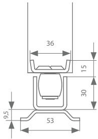
Vloergeleiding optie 2
