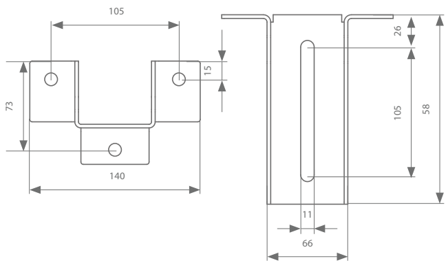
Dubbel draagstuk 121.930
