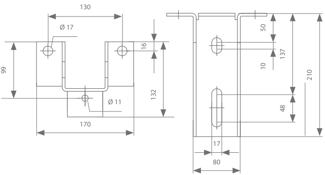
Dubbel draagstuk 141.930
