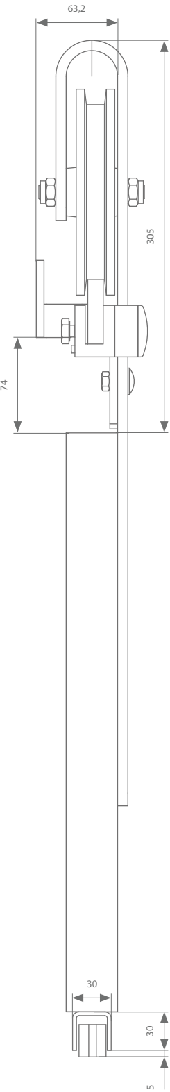
Vloergeleiding optie 1
