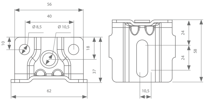
Draagstuk 121.910 121.917 (inox)
