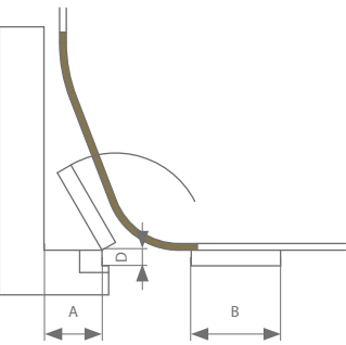
Dienstvleugel is vast aan de deurstijl
