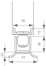
Vloergeleiding optie 2
