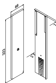
Rechts Gebruik met of zonder bekleding MOD 8245 Voor trapmontage
