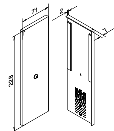
Rechts Voor MOD 8234 Voor trapmontage
