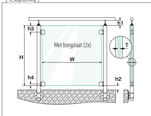
Testopstelling
