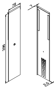
Links Voor MOD 8444 Voor trapmontage
