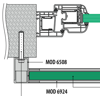
Montage op de gevel
