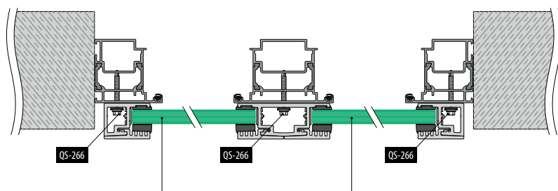
Montage met middenprofiel
