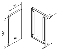
Links Voor MOD 8234
