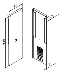
Links Voor MOD 8234 Voor trapmontage
