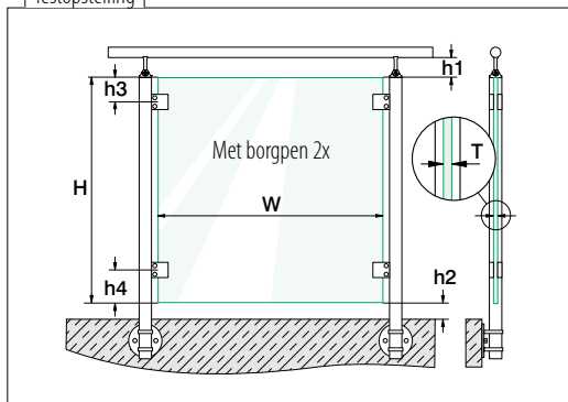
Testopstelling
