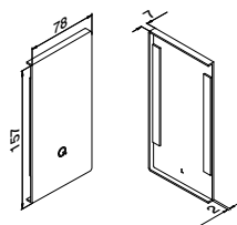
Links Voor MOD 8434
