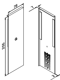
Links Voor MOD 8434 Voor trapmontage
