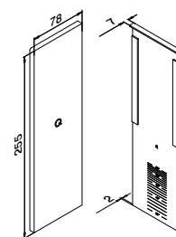
Rechts Voor MOD 8434 Voor trapmontage
