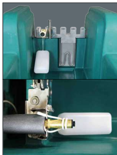
Variante I: 1x MAXIFLOW-Ventil (an Sticleitung mit Frostschutz- Heizleitung 24 V, 20 W, 2 m), 1x Zusatzheizung 24 V, 180 W
