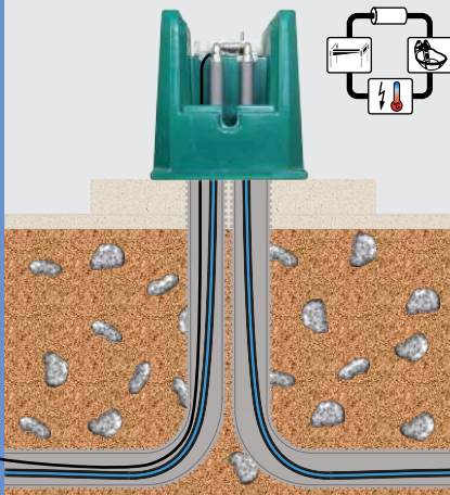
Aufbauschema für eine 1"-Ringleitung. Für Details fragen Sie bitte Ihren Fachhändler.
