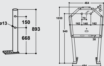
Afdeksplaat 131.6090
