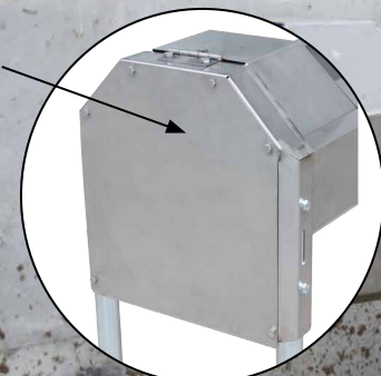
Stophouder DE LUXE: eenvoudig openen en sluiten van de afvoer boven het wateroppervlak
