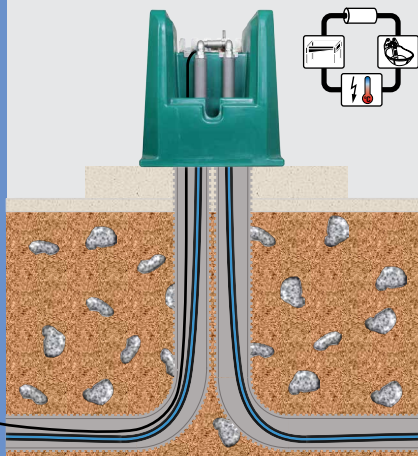
Opbouwschema voor een 1"-ringleiding. Voor details kunt u uw dealer informeren.
