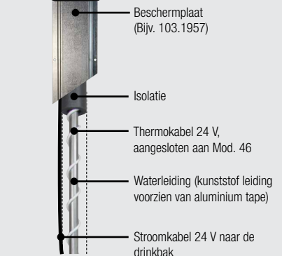
101.1405 Ventiel-verwarming 24 V, 5 W
