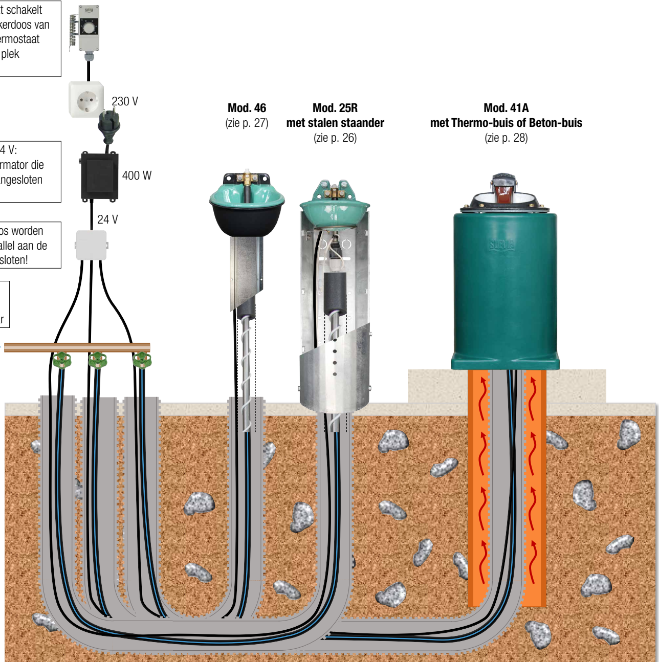
Opbouwschema met optimale presentatie, zonder isolatie van de buis. Voor details kunt u uw dealer raadplegen. Houdt de montageaanleiding in acht!
