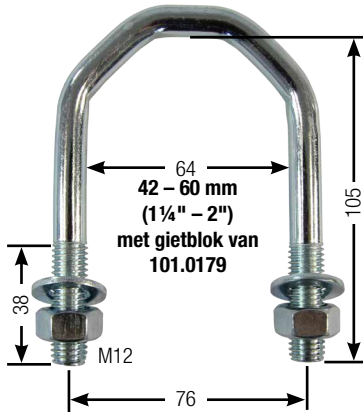
102.0177 Draadbeugel 42 – 60 mm (1¼" – 2") verzinkt (voor bijv. Draadbeugelset 101.0179 met gietblok)
