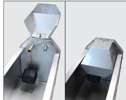
130.6181 Volume-drinkbak 3,15 m met: - 131.0726 Vlotter Mod. 726 - 131.0775 Vlotterafdekking
