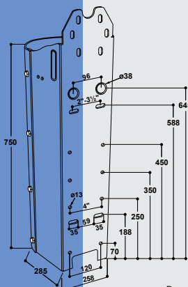
101.0456 (voor Mod. 25R)
