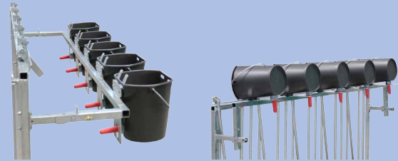
131.1762 Houder voor 5 speenemmers, opklapbaar en vergrendelbaar
