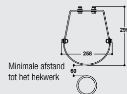
100.1239 + Toebehoren voor ringleiding met verwarmingselement
