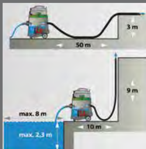
EPS 50 Förderschema
