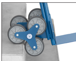
Driearmige wielster TK1325 | TK1326
