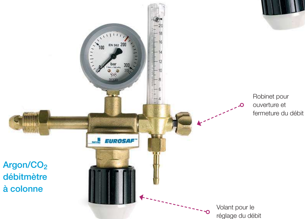
Argon/CO 2 mano-débitmètre
